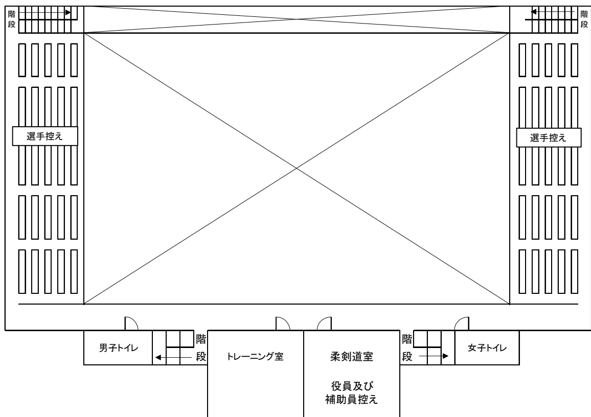
2階 配置図
