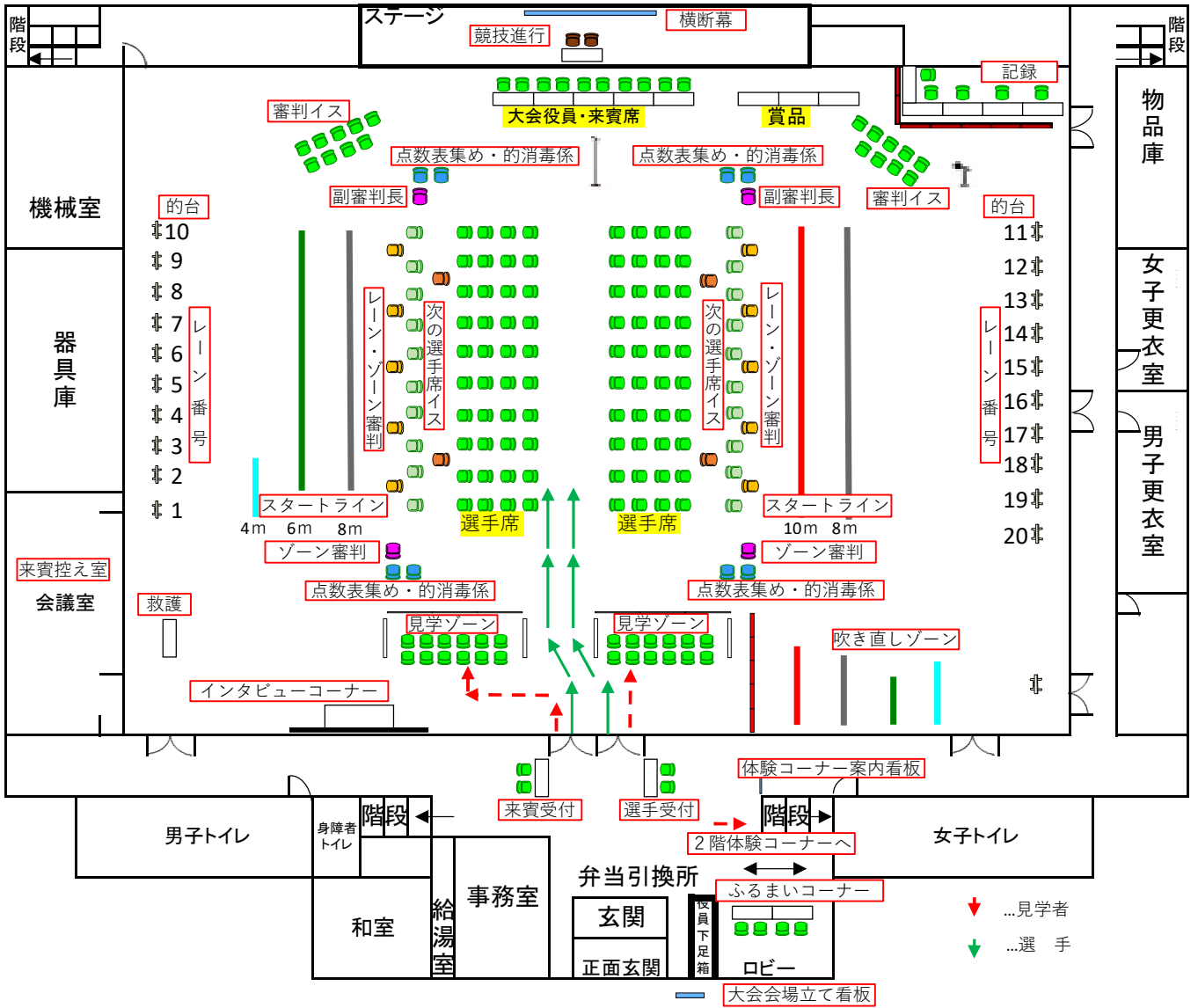
1階 配置図
